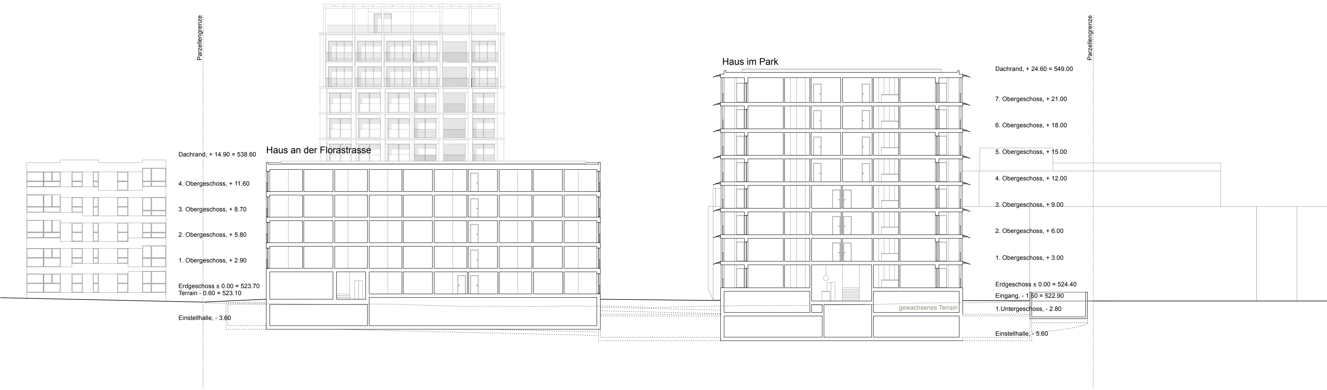
Schnitt Nord-Süd
